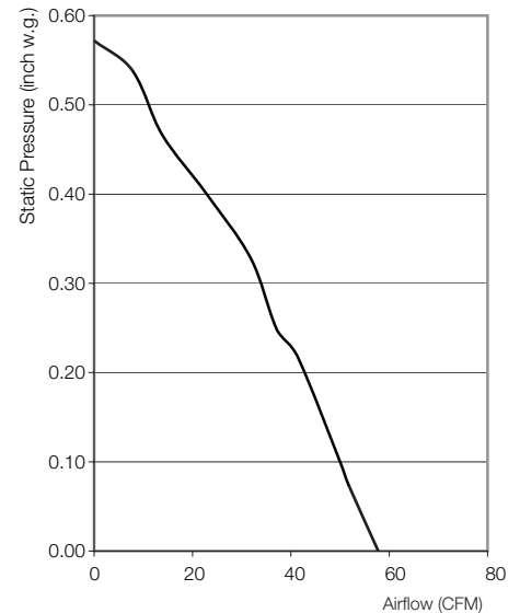
Fan Curve FV-05VS1
